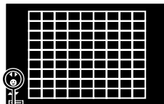
Метод выбора
