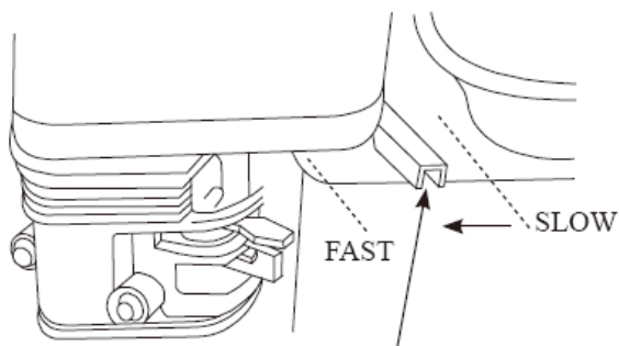
РЫЧАГ ДРОССЕЛЯ
